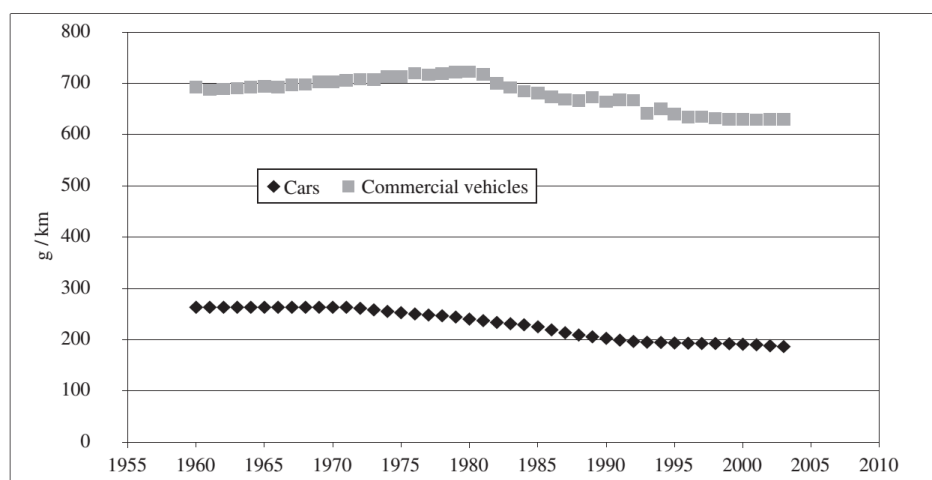
Fig. 9 Emissioni CO 2 in Germania. Fonte: SRU (2005)
