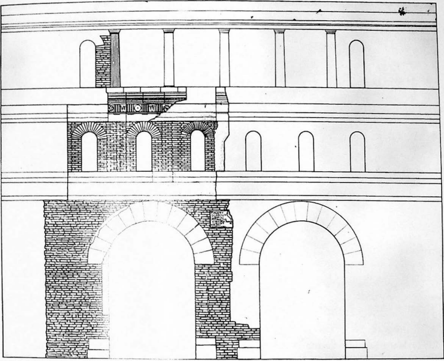
Fig. 1. VERONA. Prospetto interno della Porta Leoni, fase repubblicana (dis. Soprint. Archeologica del Veneto).
